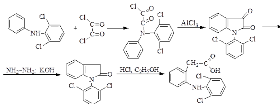
Рис. 2 – Синтез диклофенака
