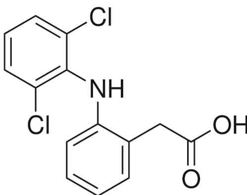
Рис. 1 – Формула диклофенака
